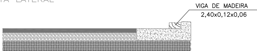
VISTA LATERAL
